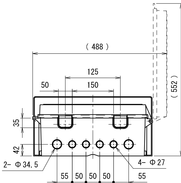
底面図 1/8
